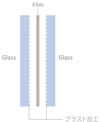
<インナーブラストガラスの構造>
